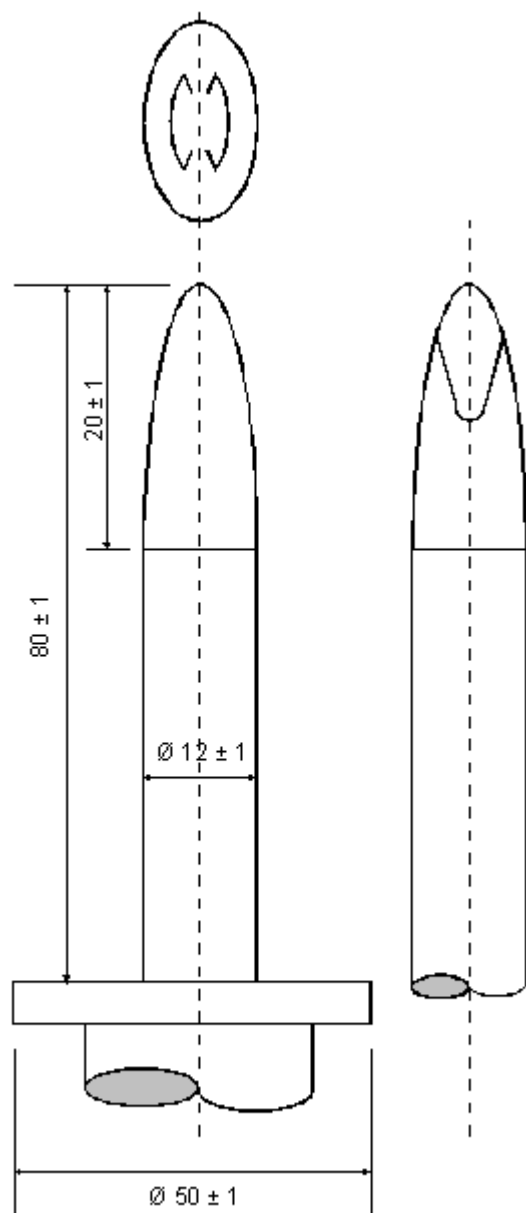
Figura 2. Dedo de prueba rígido Dimensiones en mm
