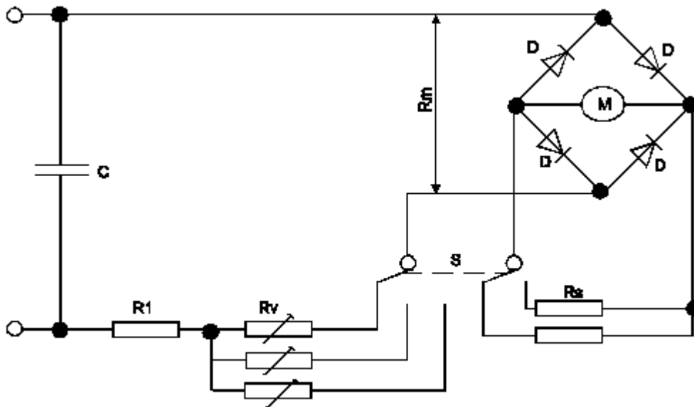
Figura 1 Circuito para medir corriente de fuga
