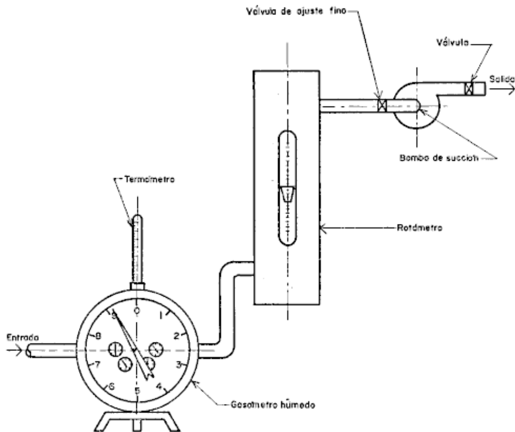
FIGURA 1.- SISTEMA DE CALIBRACION DEL ROTAMETRO
