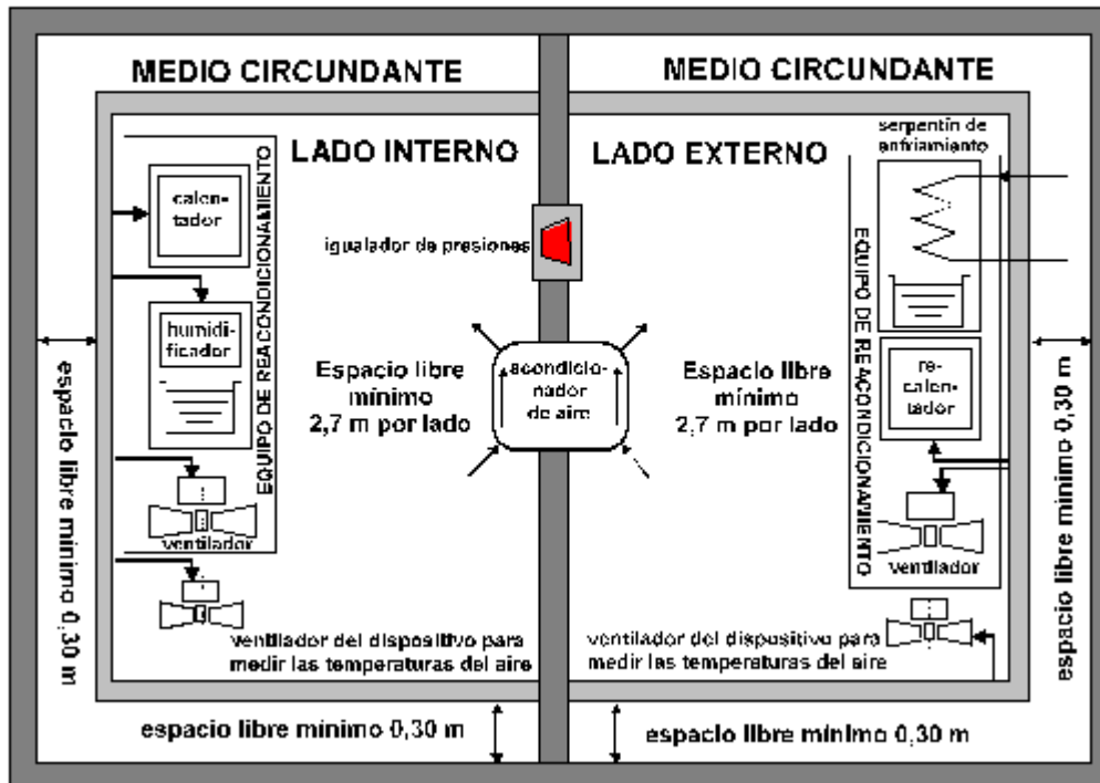
Figura 1. Calorímetro de cuarto tipo ambiente balanceado
