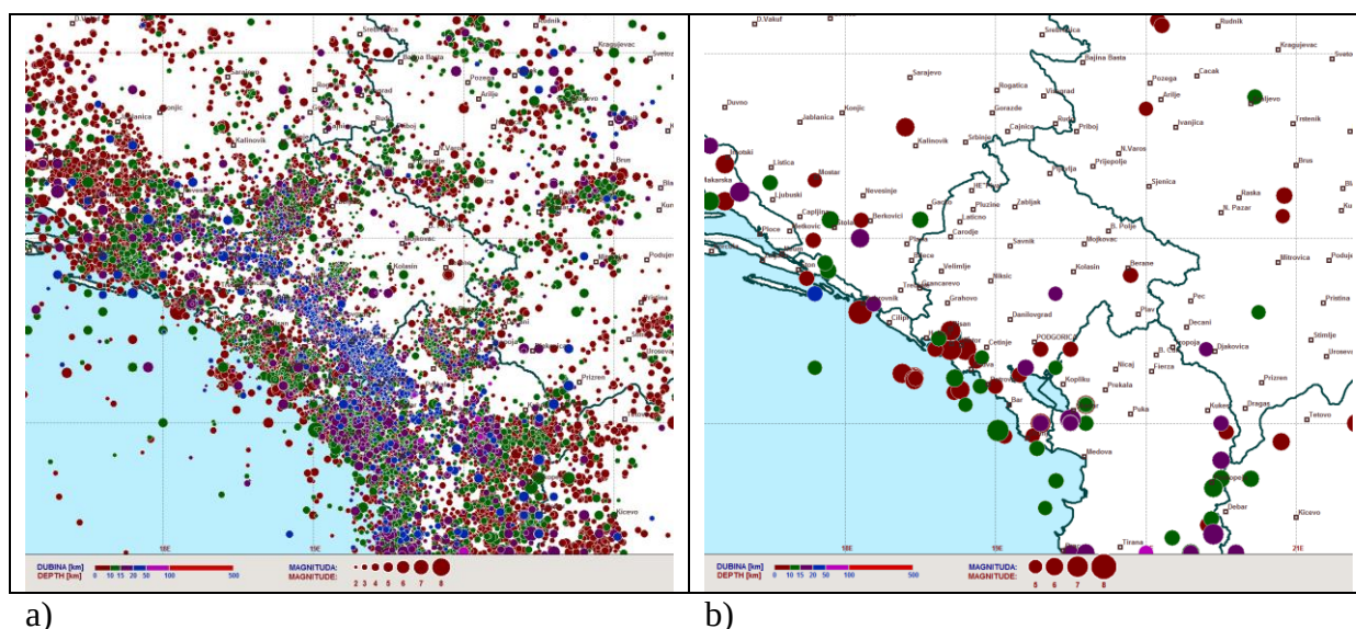
Slika 1: a) Karta epicentara zemljotresa u Crnoj Gori i neposrednom okruženju u periodu 1944-2016 godine. b) Izdvojeni snažniji zemljotresi ( M > 5 ). Prema datoj legendi veličina simbola na karti indicira njegovu jačinu dok boja simbola označava dubinu žarišta.
