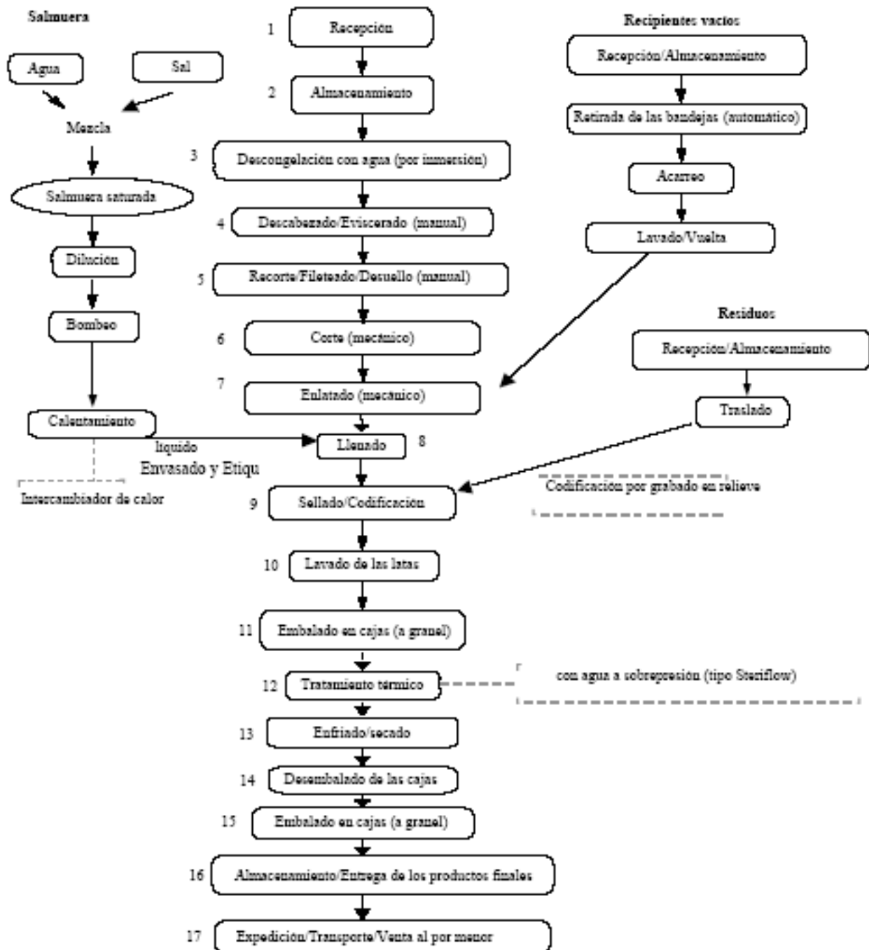
Figura 5.2 Ejemplo de diagrama de flujo para una cadena de elaboración de atún en conserva
