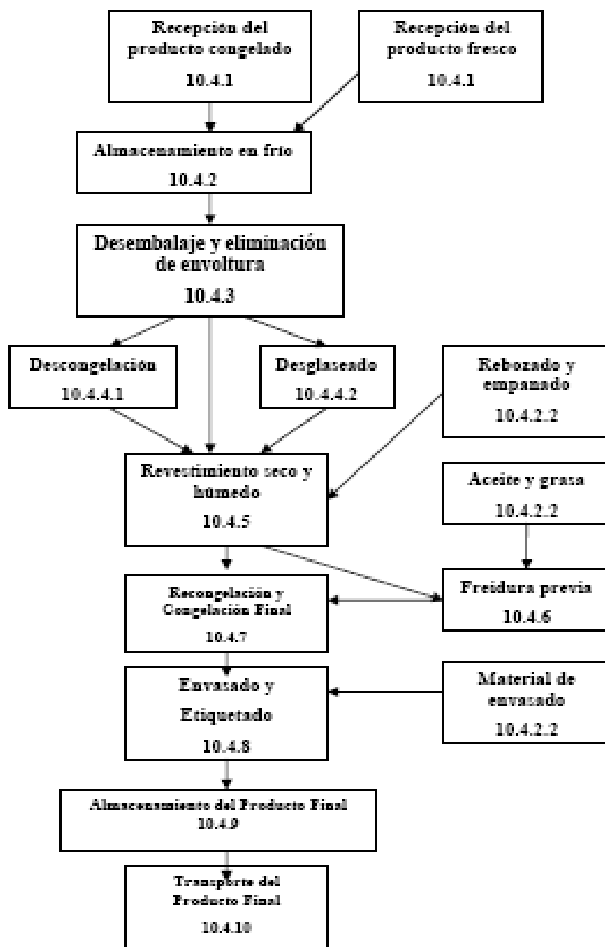
Figura 10.2 Ejemplo de Diagrama de Flujo de la Línea de Elaboración de Mariscos Moluscosoides Revestidos
