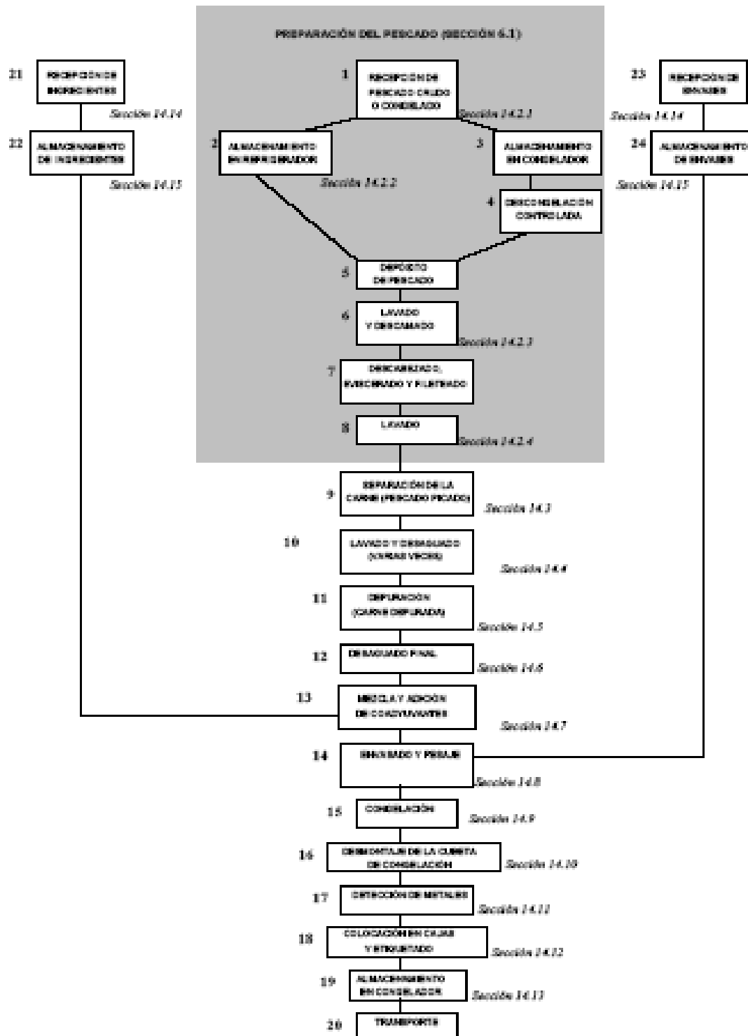
Figura 9.1 Ejemplo de diagrama de flujo para un proceso de producción de surimi congelado
