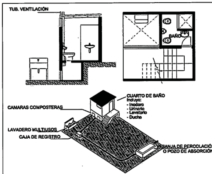
Ilustración 38: Vista en corte y planta de una U.B.S. con compostera
