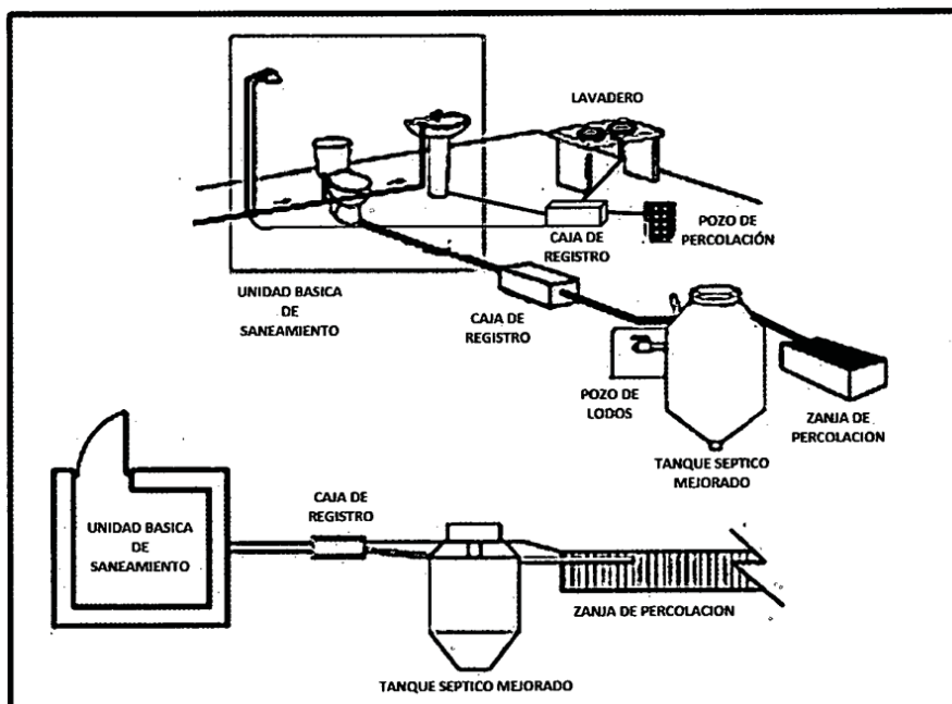
Ilustración 35: Gráfico de U.B.S-A.H. con tanque séptico mejorado
