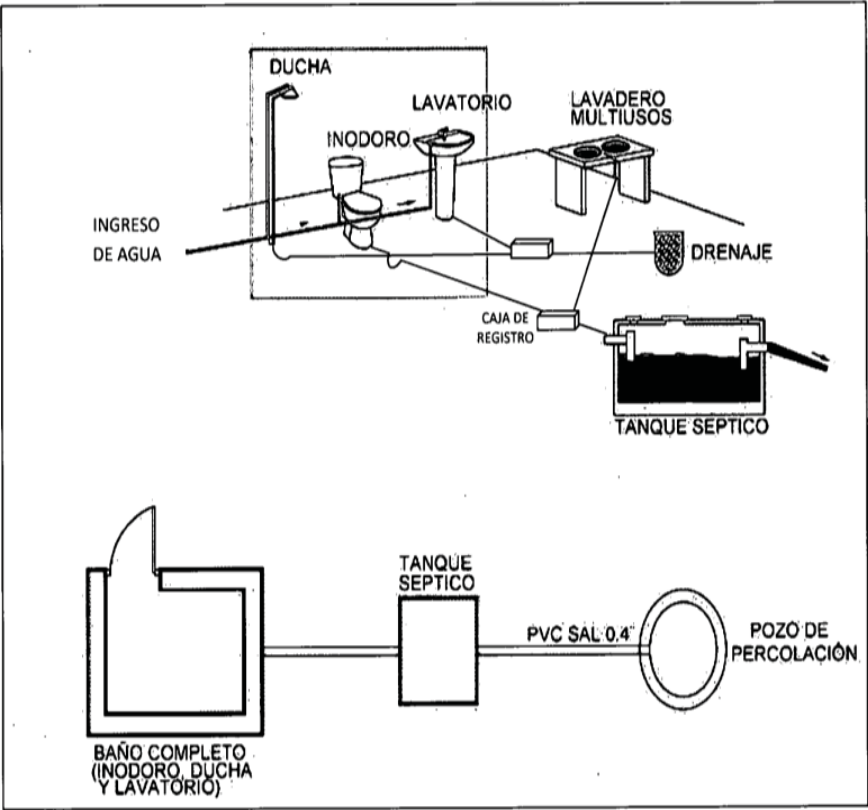
Ilustración 34: Esquema de las tipologías referentes a la U.B.S con tanque séptico
