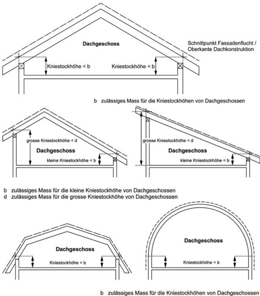
Figur 6.3 Dachgeschosse
