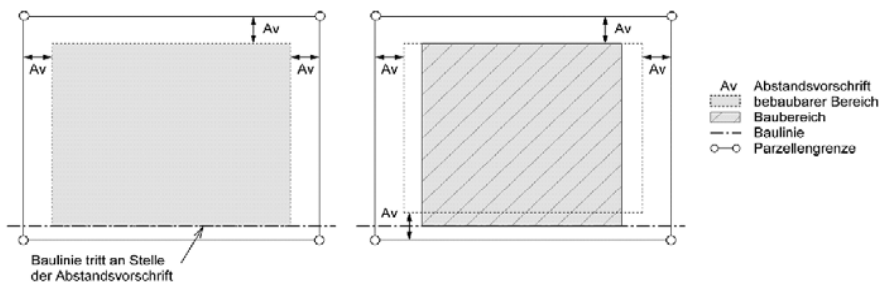
Figur 7.1 - 7.3 Abstände und Abstandsbereiche
