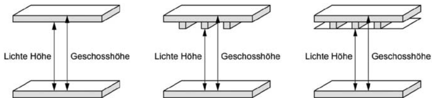
Figur 5.4 Lichte Höhe
