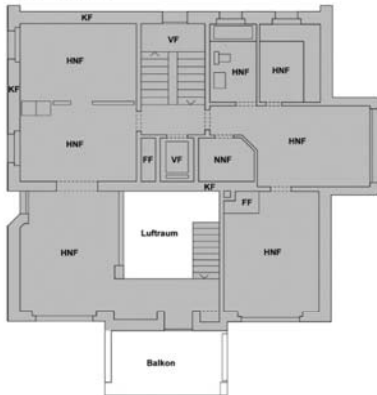
Grundriss 1. Obergeschoss:
