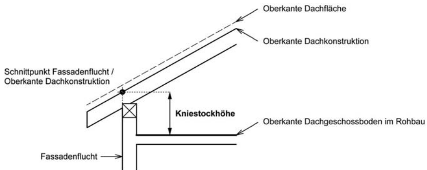
Figur 5.3 Kniestockhöhe
