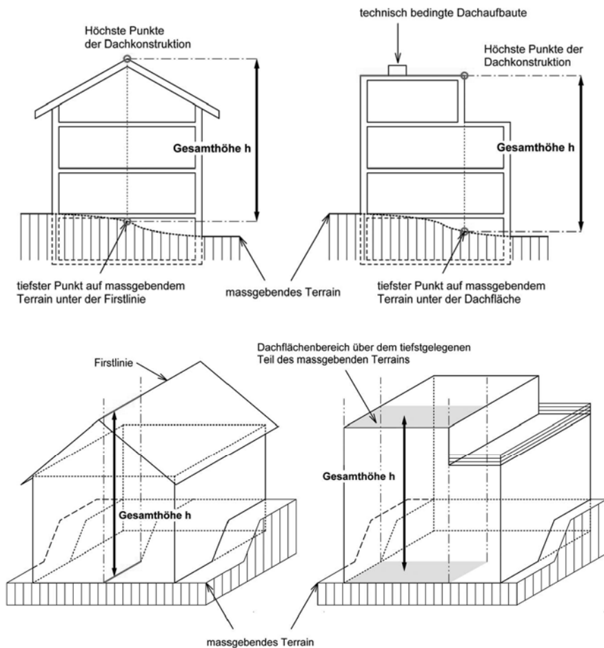
Figur 5.1 Gesamthöhe
