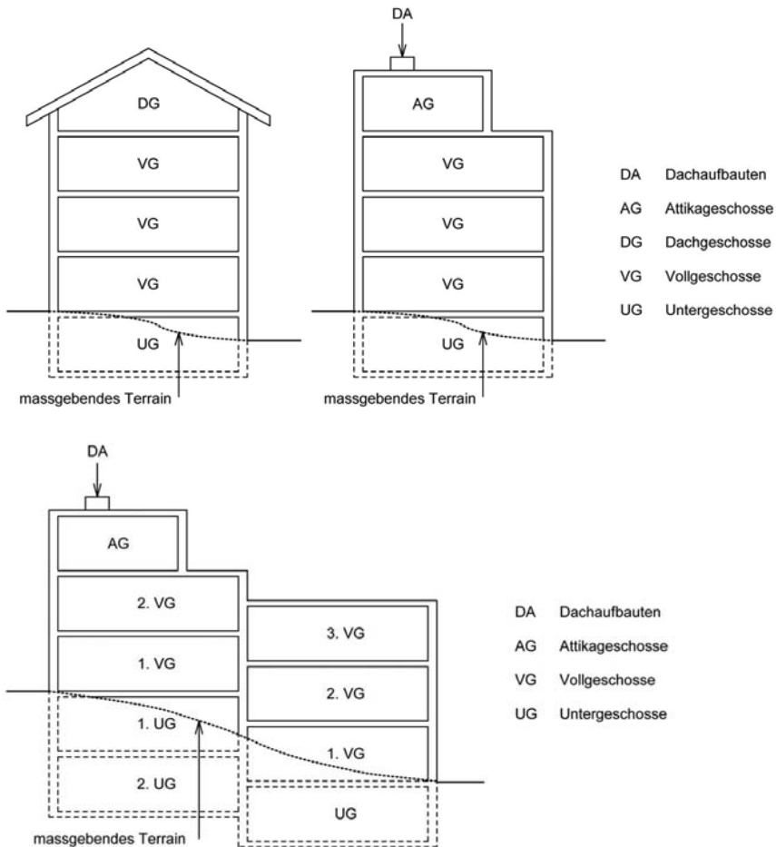
Figur 6.1 Geschosse und Geschosszahl
