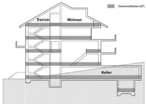
Schnitt:
