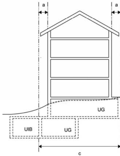
Figur 6.2 Untergeschosse
