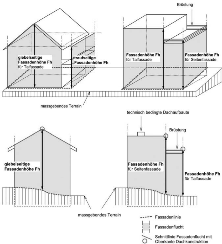
Figur 5.2 Fassadenhöhe
