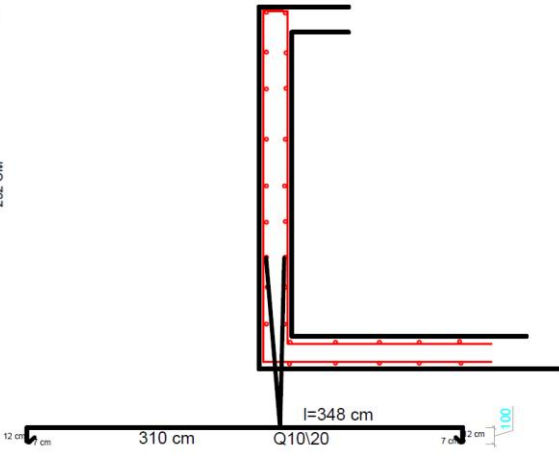
G-G kesiti donatı şeması
