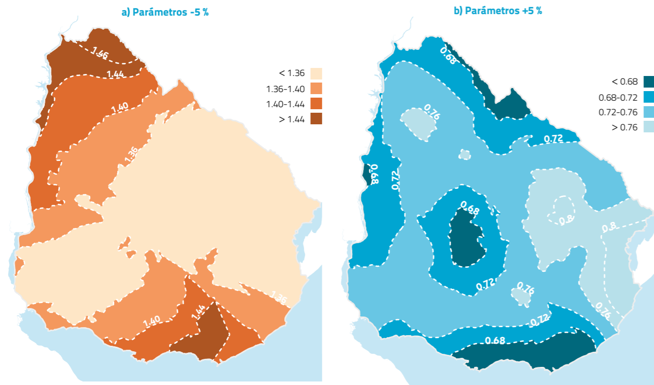
Figura 9.19 | Relación para la probabilidad de ocurrencia de rachas secas mayores a 30 días en el período cálido entre las series sintetizadas por el generador de tiempo en escenarios (+/- 5 %) y con parámetros climatológicos
