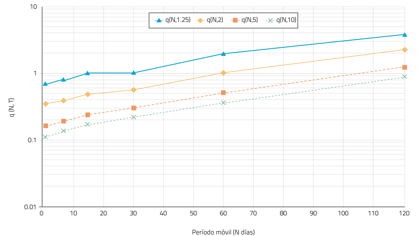
Figura 5.9 | Caudales mínimos específicos en N días consecutivos con período de retorno T años Estación N° 59,1-Paso Pache-Río Santa Lucía (1980 - 2010)
